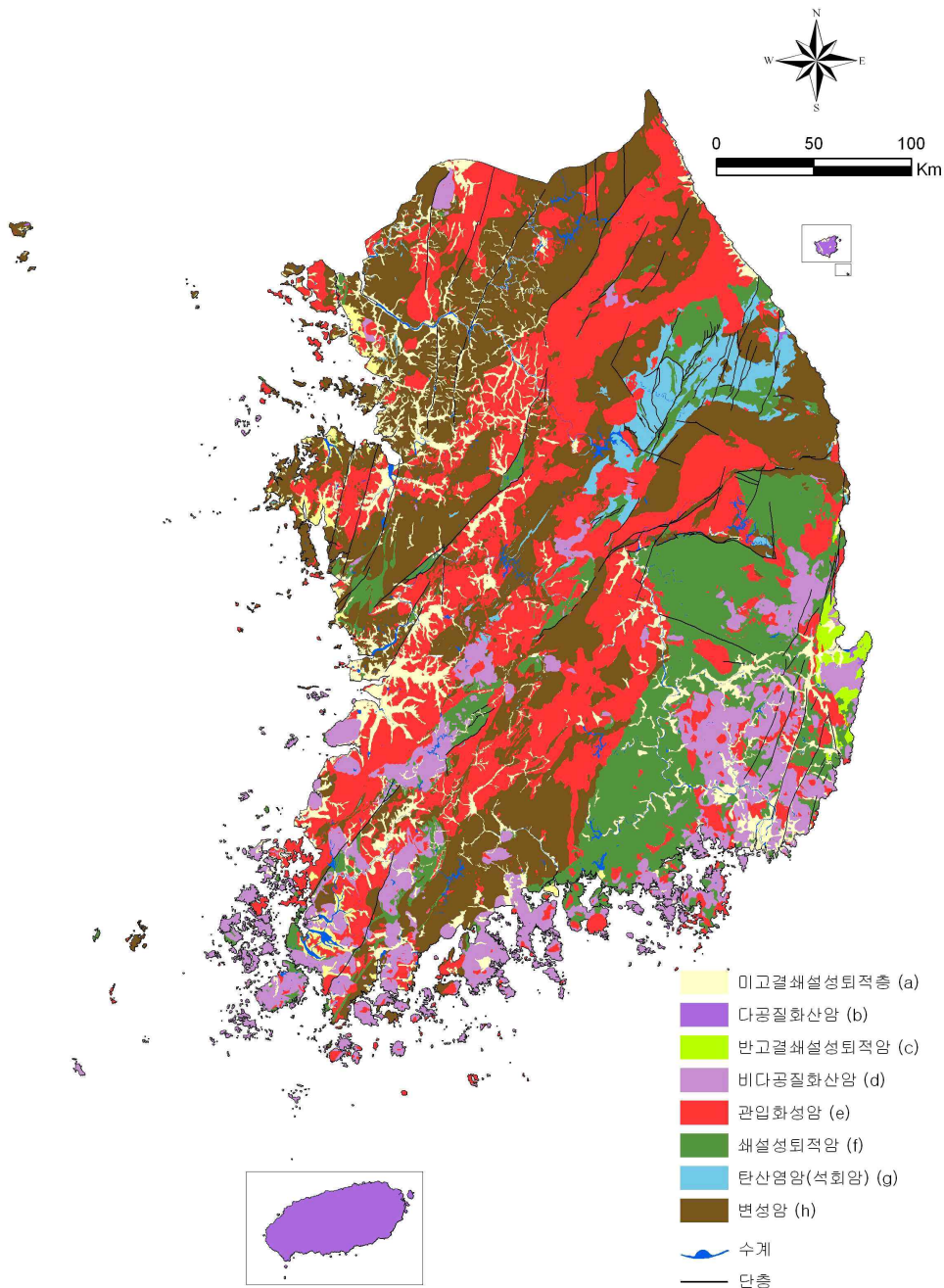
【전국 수문지질도】
